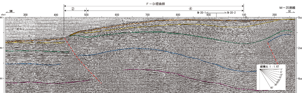
M-20測線【F-D褶曲群主部】
