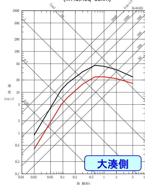
— F-B断層による地震(M6.8, Xeq=14km) — 米山沖断層～高田平野西縁断層帯による地震 (M7.1, Xeq=35km)
