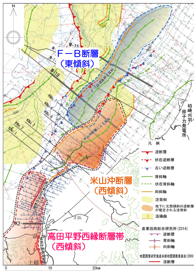
— F-B断層による地震(M6.8, Xeq=14km) — 米山沖断層～高田平野西縁断層帯による地震 (M7.1, Xeq=34km)
