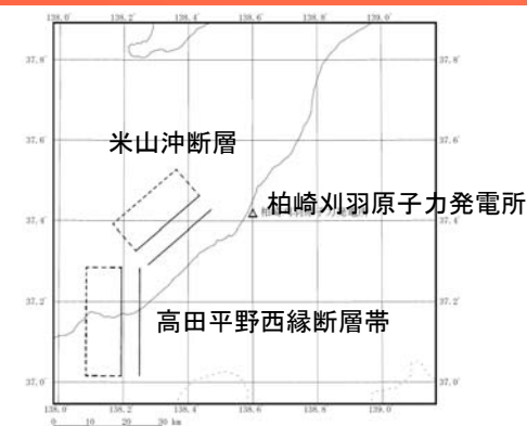
— F-B断層による地震(M6.8, Xeq=14km) — 米山沖断層～高田平野西縁断層帯による地震 (M7.1, Xeq=35km)
