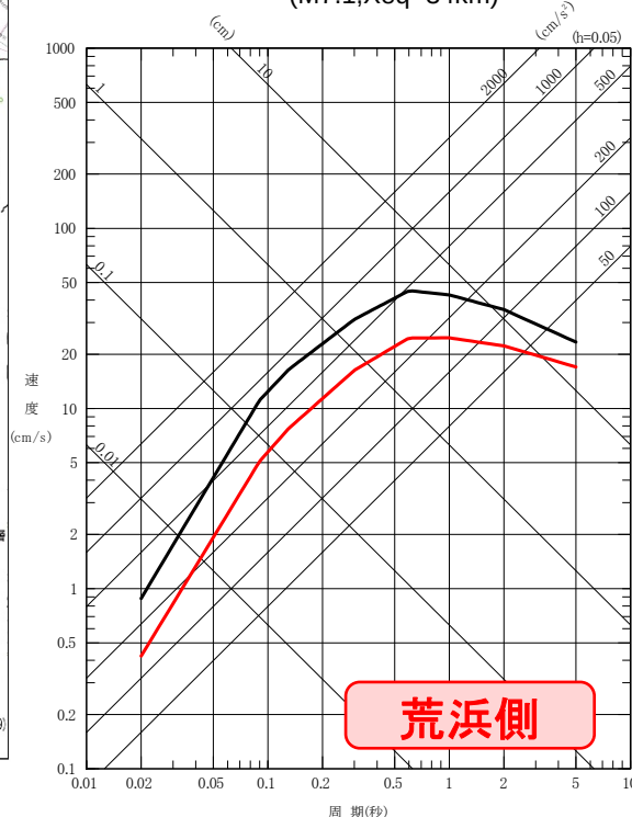
— F-B断層による地震(M6.8, Xeq=14km) — 米山沖断層～高田平野西縁断層帯による地震 (M7.1, Xeq=34km)
