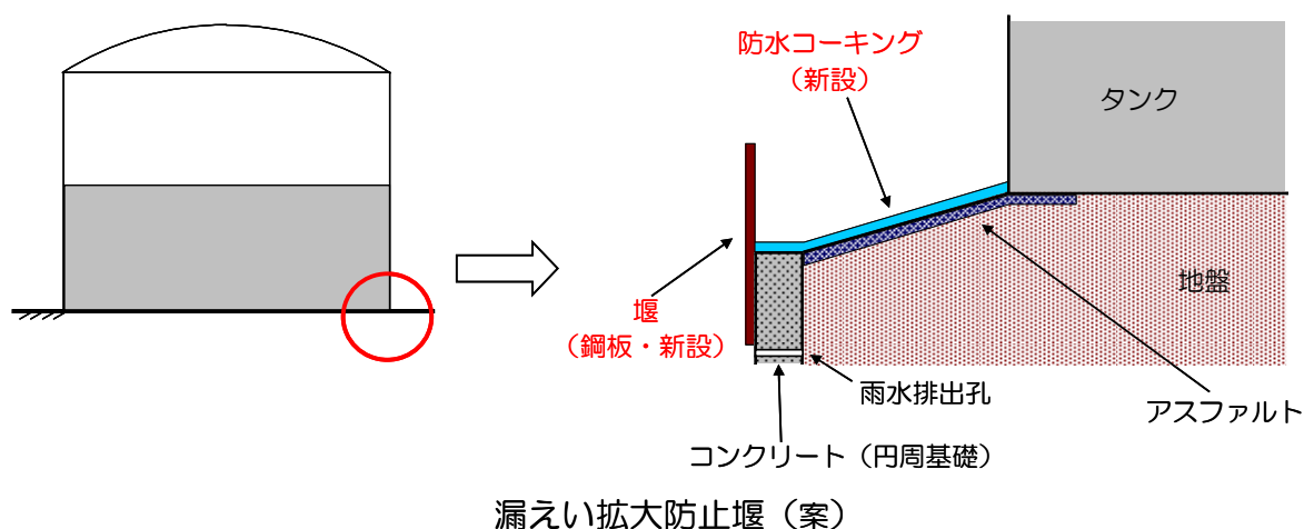
図－３ No.1 ろ過水タンク廻り堰構造概要
