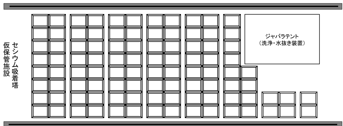
図ー４ 使用済セシウム吸着塔仮保管施設
