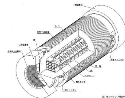
NFT-32B型外観図 (扱いを検討中)
