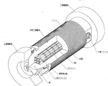
NFT-12B型外観図
