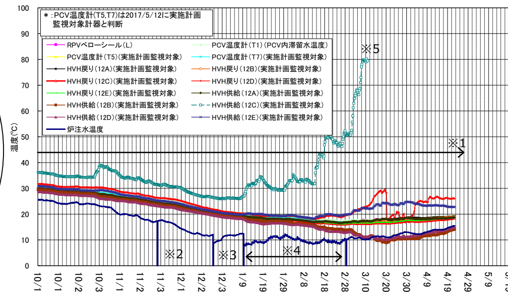
1号機 D/W雰囲気温度 (10/1～4/22)
