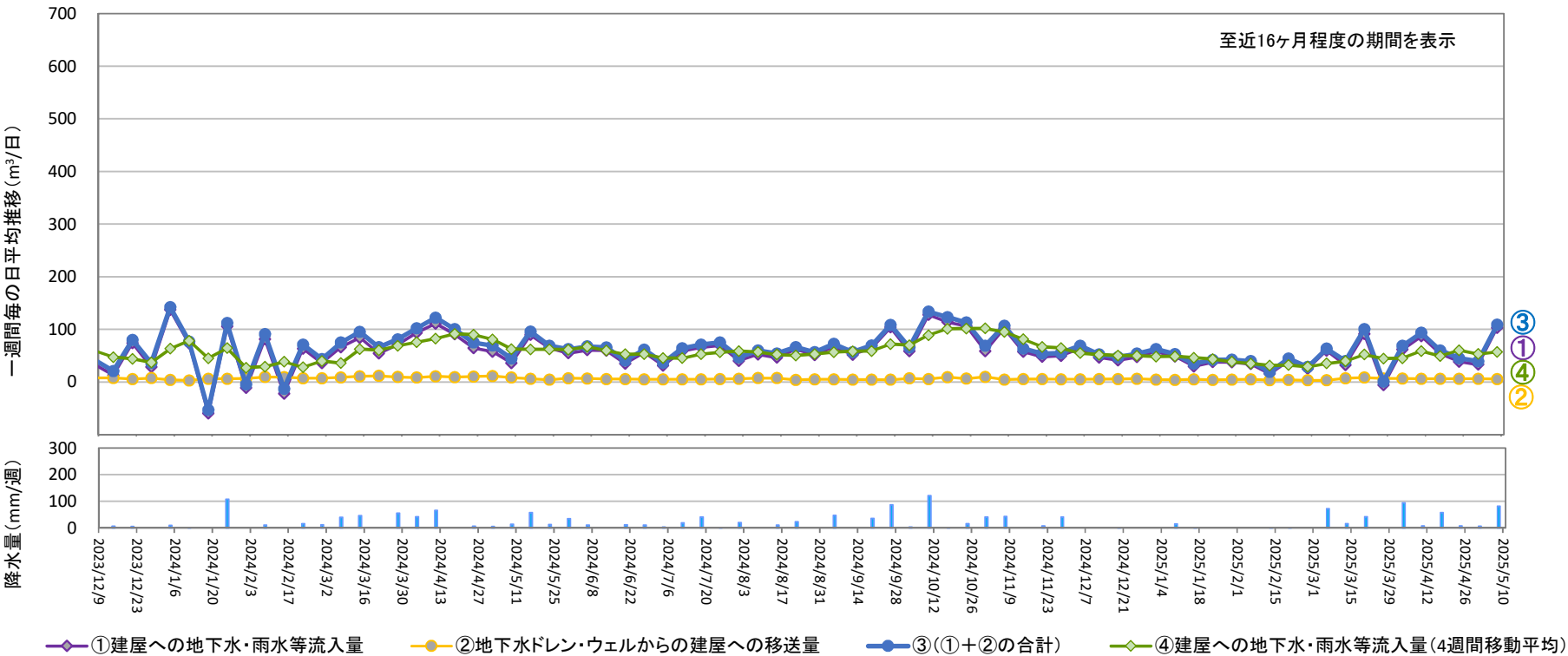
地下水ドレンからタービン建屋への移送量 ( 2025年5月1日 ~ 2025年5月7日 ) [m³／日]
