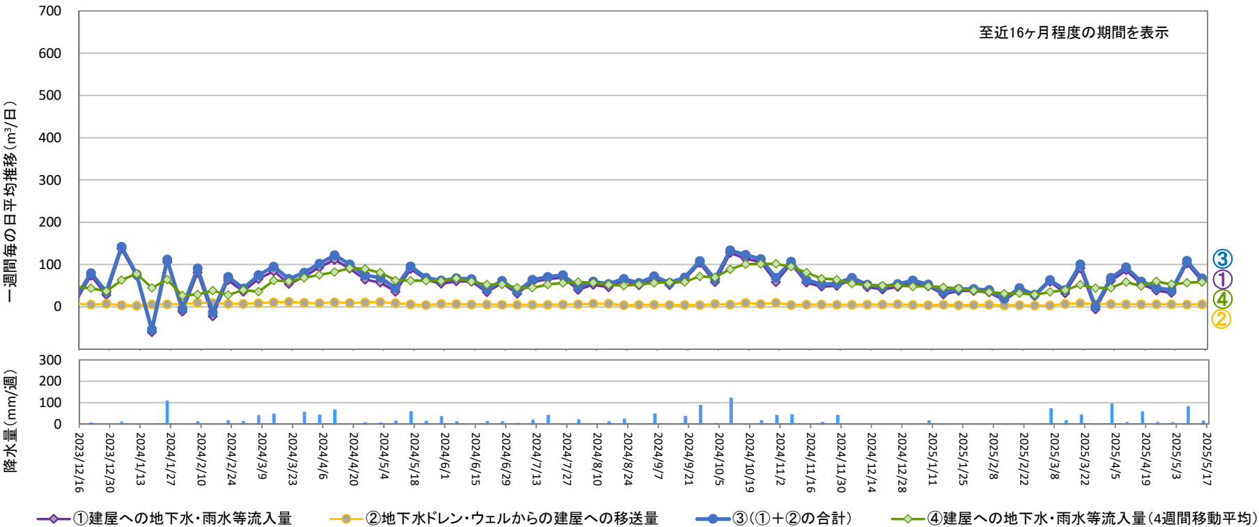
地下水ドレンからタービン建屋への移送量 ( 2025年5月8日 ~ 2025年5月14日 ) [m³/日]
