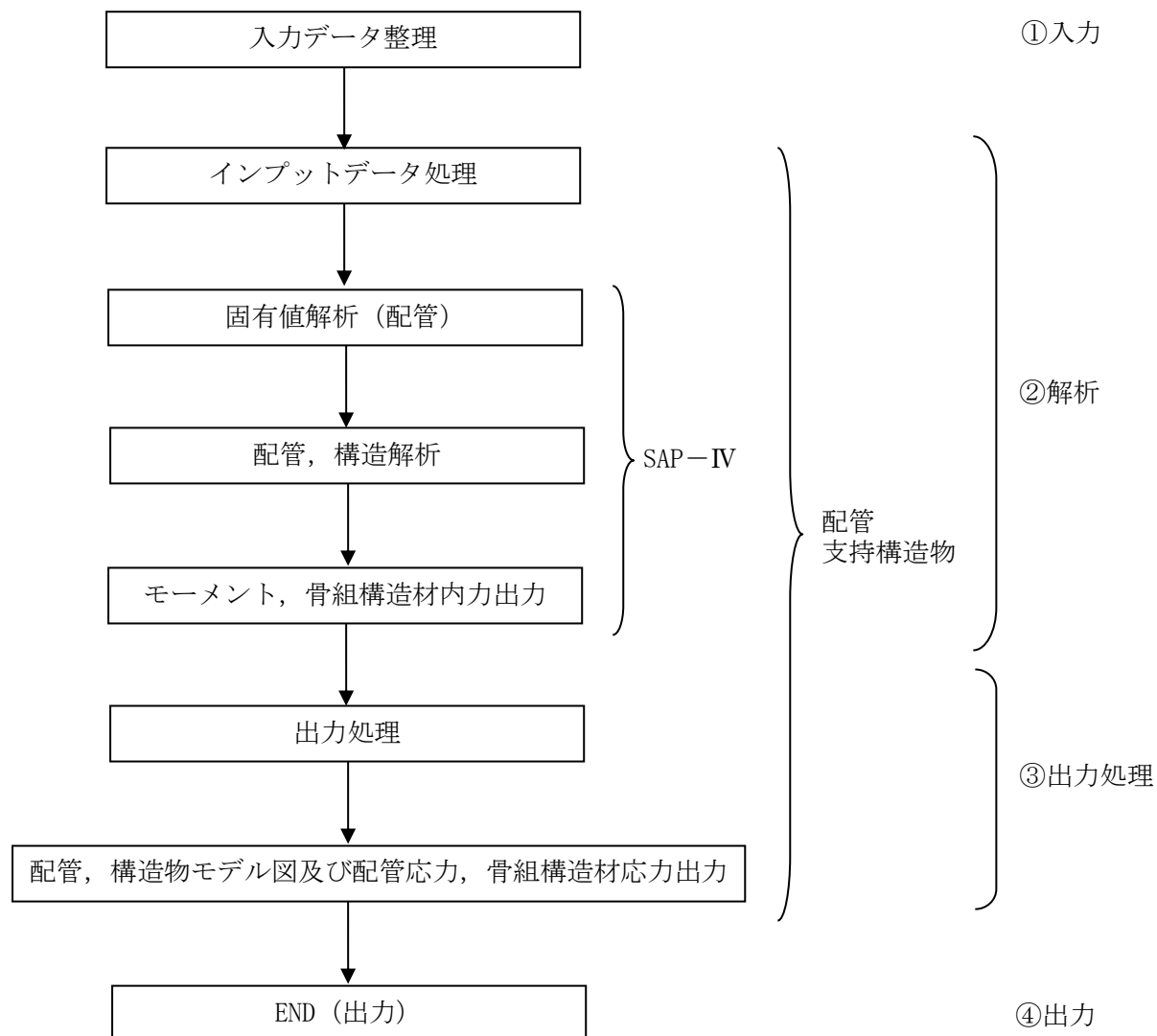
図 1-1 計算フロー
