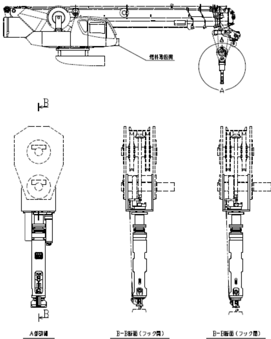
図一 2 燃料把握機 外形図
