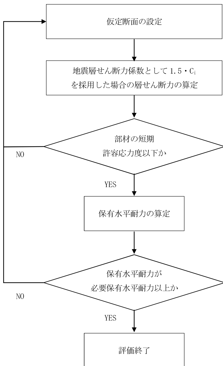
図ー9 Bクラス施設としての建屋の耐震安全性評価手順
