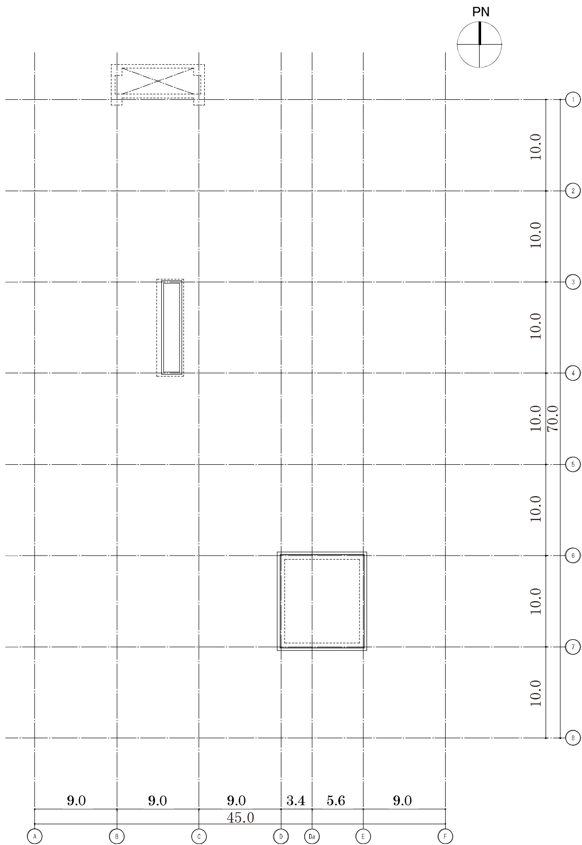
图一6 屋根平面图 (G. L. +29.30) (单位 : m)
