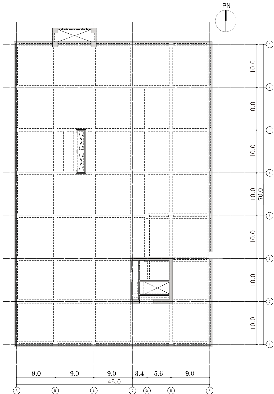
图一5 屋上階平面図 (G. L. +24. 30) (单位 : m)
