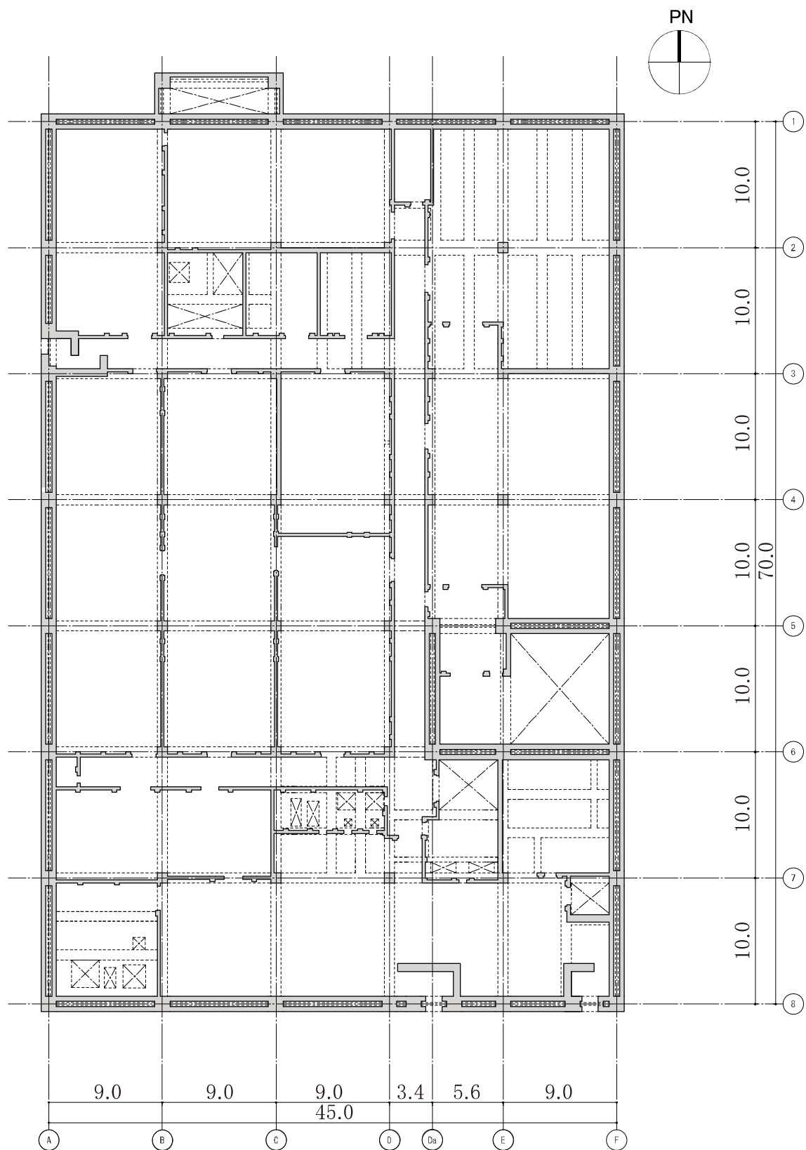
图一3 2階平面図 (G.L. +8.80) (単位 : m)
