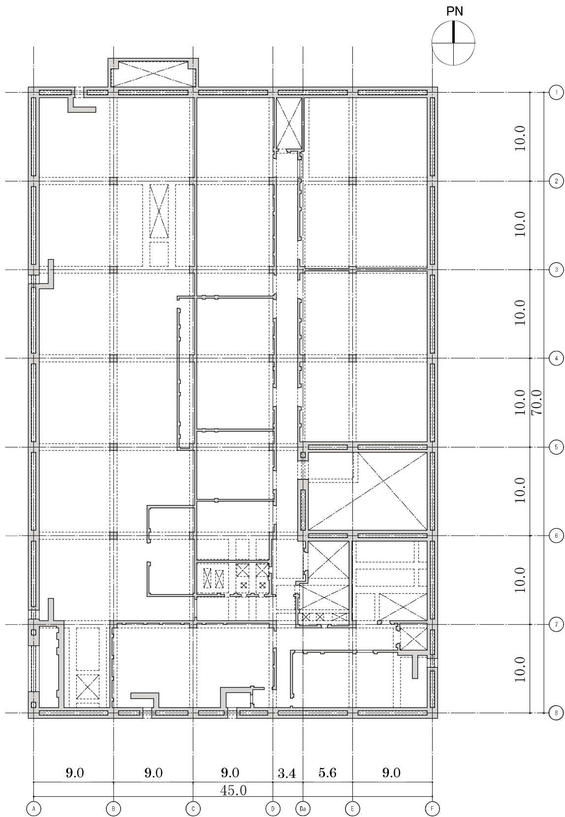
图-4 3 階平面図 (G. L. +15.80) (単位 : m)
