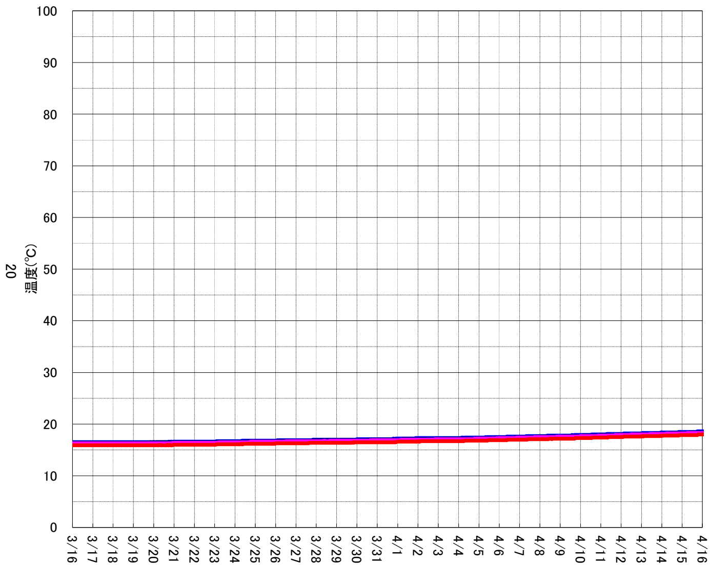
1号機 RPV周辺温度計(下部)
