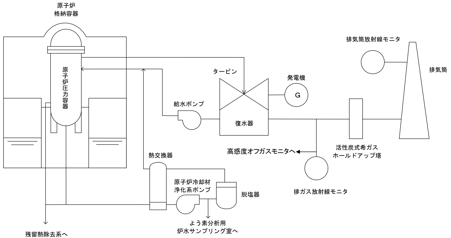
7 号 機 系 統 概 略 図
