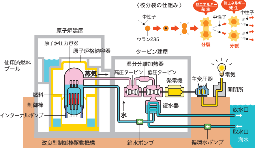
※改良型沸騰水型原子炉（6～7号機）の例
